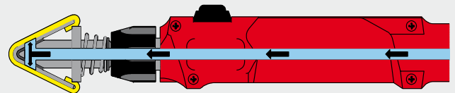
/ Puhdistuskynään kiinteä elektrolyytinsyöttö; virtausnopeutta säädellään tarkasti joko manuaalisesti tai automaattisella syöttötoiminnolla.
